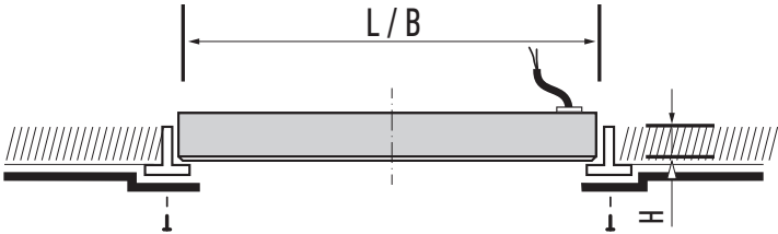
Рис. 1 Схема встраиваемого монтажа светильника PPL SPEC
